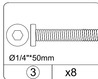
Bolt Boulon TGF0170
