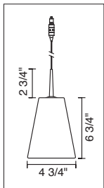
BLING II LED DOWN 222 169(bz,ch,mc) 222 174(bz,ch,mc) 222 179(bz,ch,mc) 222 843(bz,ch,mc) 222 844(bz,ch,mc) 222 845(bz,ch,mc)
