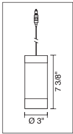
SILVA LED DOWN 222 711(bz,ch,mc) 222 712(bz,ch,mc) 222 713(bz,ch,mc) 222 714(bz,ch,mc) 222 715(bz,ch,mc) 222 716(bz,ch,mc)
