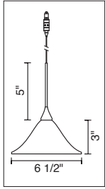
BELLA LED DOWN 222 091(bz,ch,mc) 222 092(bz,ch,mc) 222 094(bz,ch,mc) 222 096(bz,ch,mc) 222 099(bz,ch,mc)
