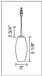
CIRO MINI LED DOWN 222 830(bz,ch,mc) 222 831(bz,ch,mc) 222 832(bz,ch,mc) 222 833(bz,ch,mc)
