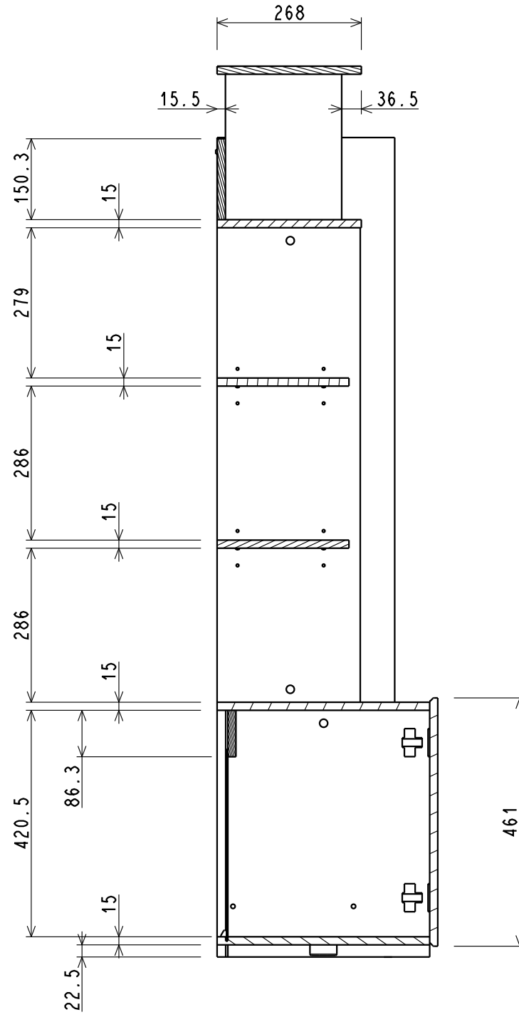
COUPE G-G
