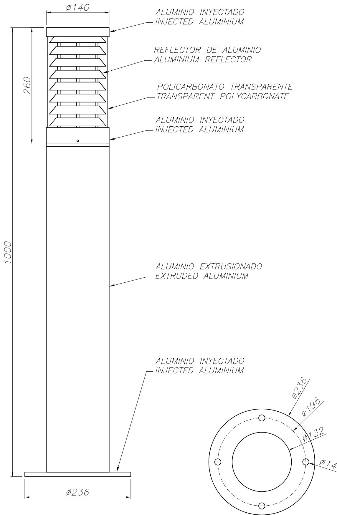
PLANTILLA DE INSTALACION INSTALLATION TEMPLATE
