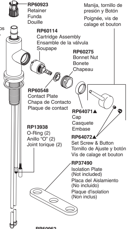
RP50952 Cut -To - Fit Plastic Sleeves Casquillos cortados a la medida Bagues d'extrémité pour tubes coupés
