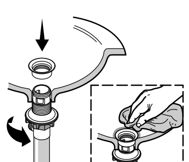
Stopper Bolt Boulon d'arrêt Perno del obturador
