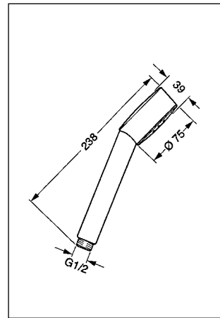
Handbrause, DN 15 Hansadesigno
