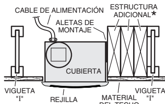
CUBIERTA MONTADA EN CUALQUIER LUGAR ENTRE LAS VIGUETAS Se requiere una estructura adicional para las aletas de montaje.
